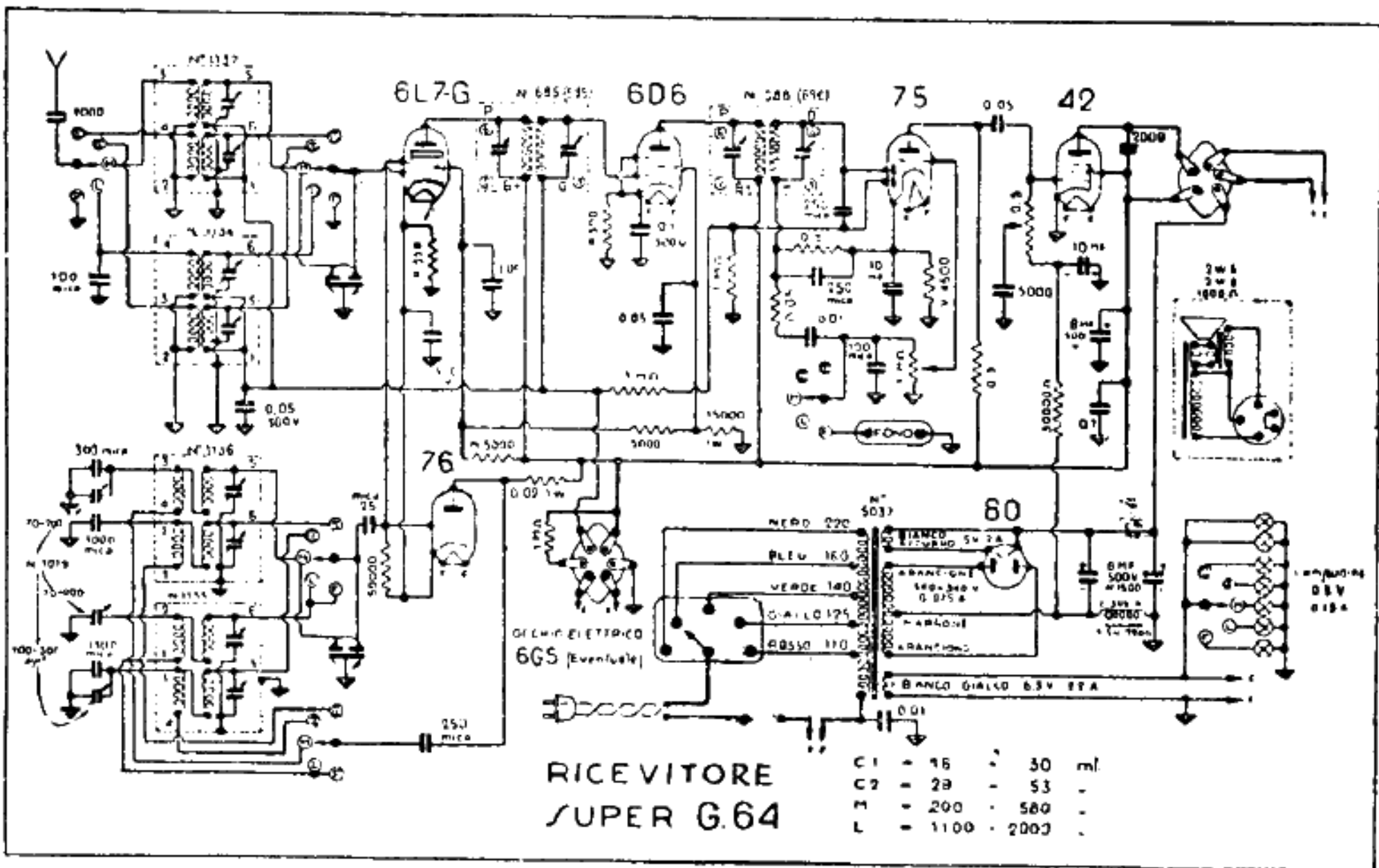
S. A. GELOSO. — Mod. G. 64. — Super a 4 gamme, da 16 a 2000 m. — Media frequenza: 467 kHz. Produzione 1937.
